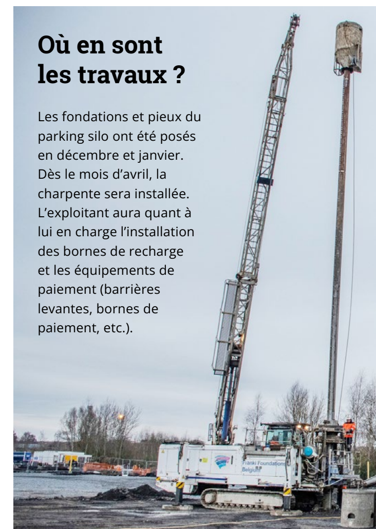
Les pieux sont forés à 23 mètres de profondeur.
